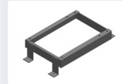
Suporte Rebaixe de Banco MB Actros Altura 50 mm após 2020.
