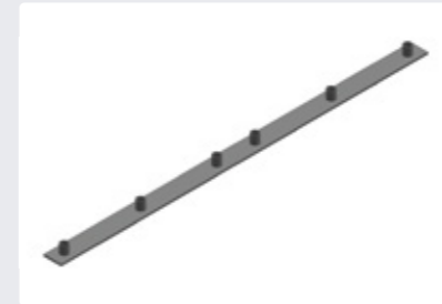
Suporte de Fixação Aparabarro Volvo FH/ NH - 627mm.
