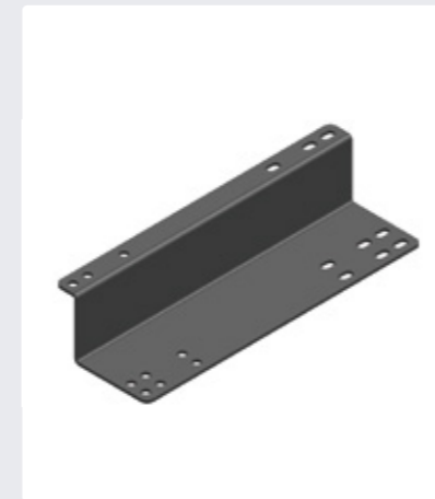
Suporte Dobrado para Fixação Caixa Ferramentas - Altura 50 mm.
